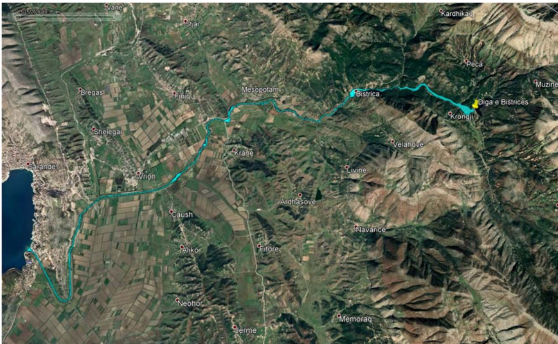
Figura C-1 Skenari 1 – Prishja e digës së Bistricës 1 me prurjen maksimale çdo 10 000 vjet 240 \text{ m}^3/\text{s}
